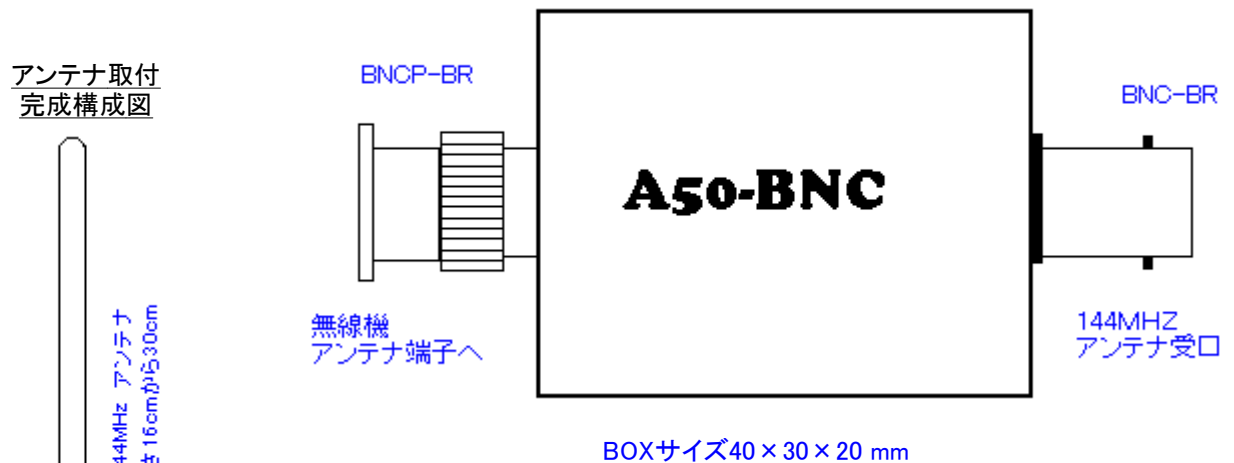
50MHz用アンテナアダプタ 完成図
